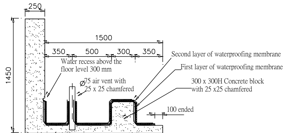
Sec A-A
