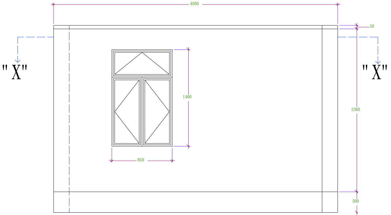
Elevation
