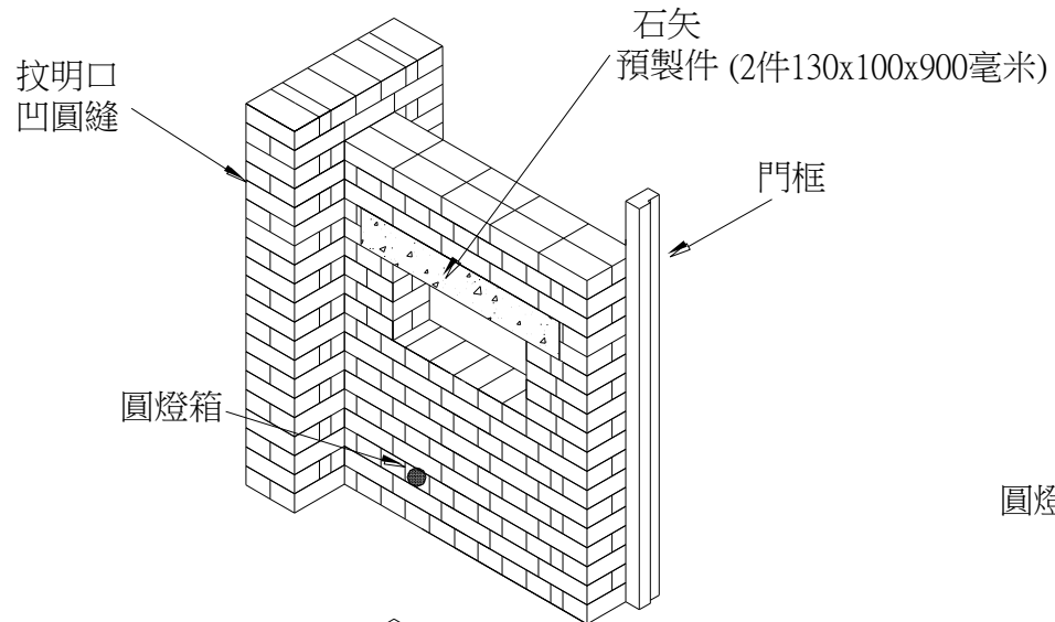
立體圖
