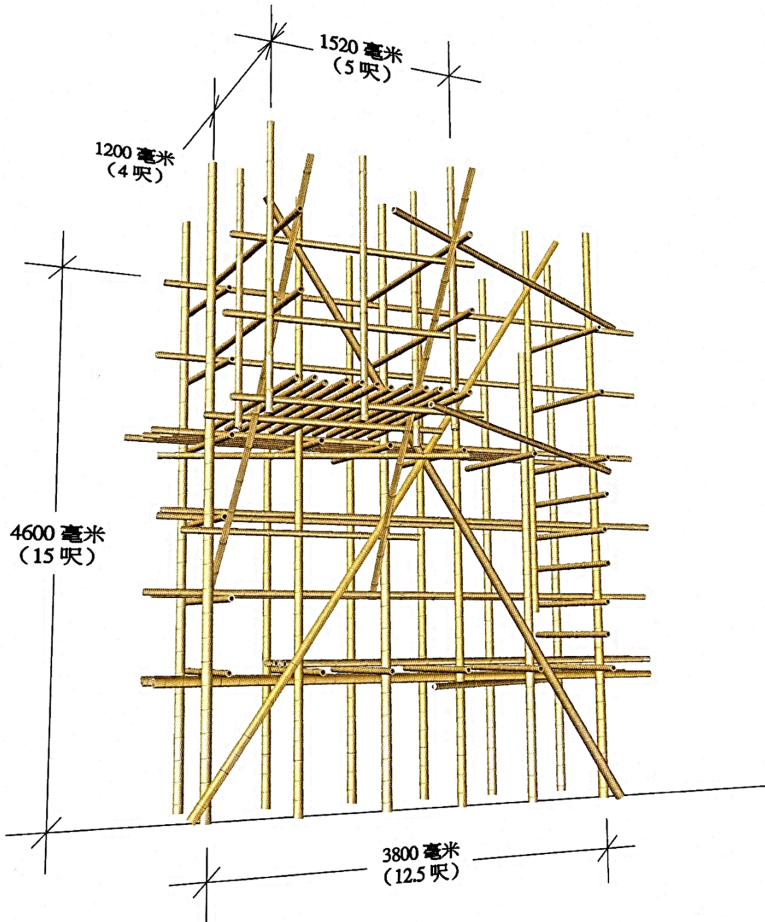
排柵、密竹橋架、挑撐棚施工圖 (不按比例)
