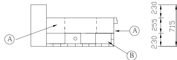
正面圖
