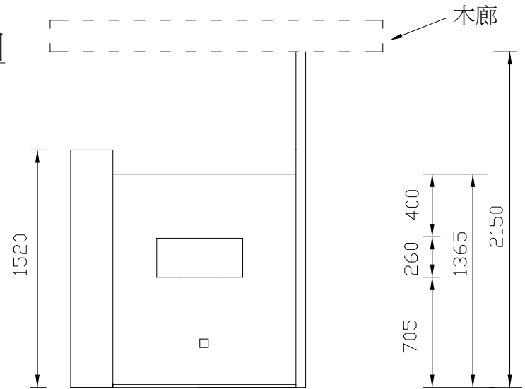
正面圖
