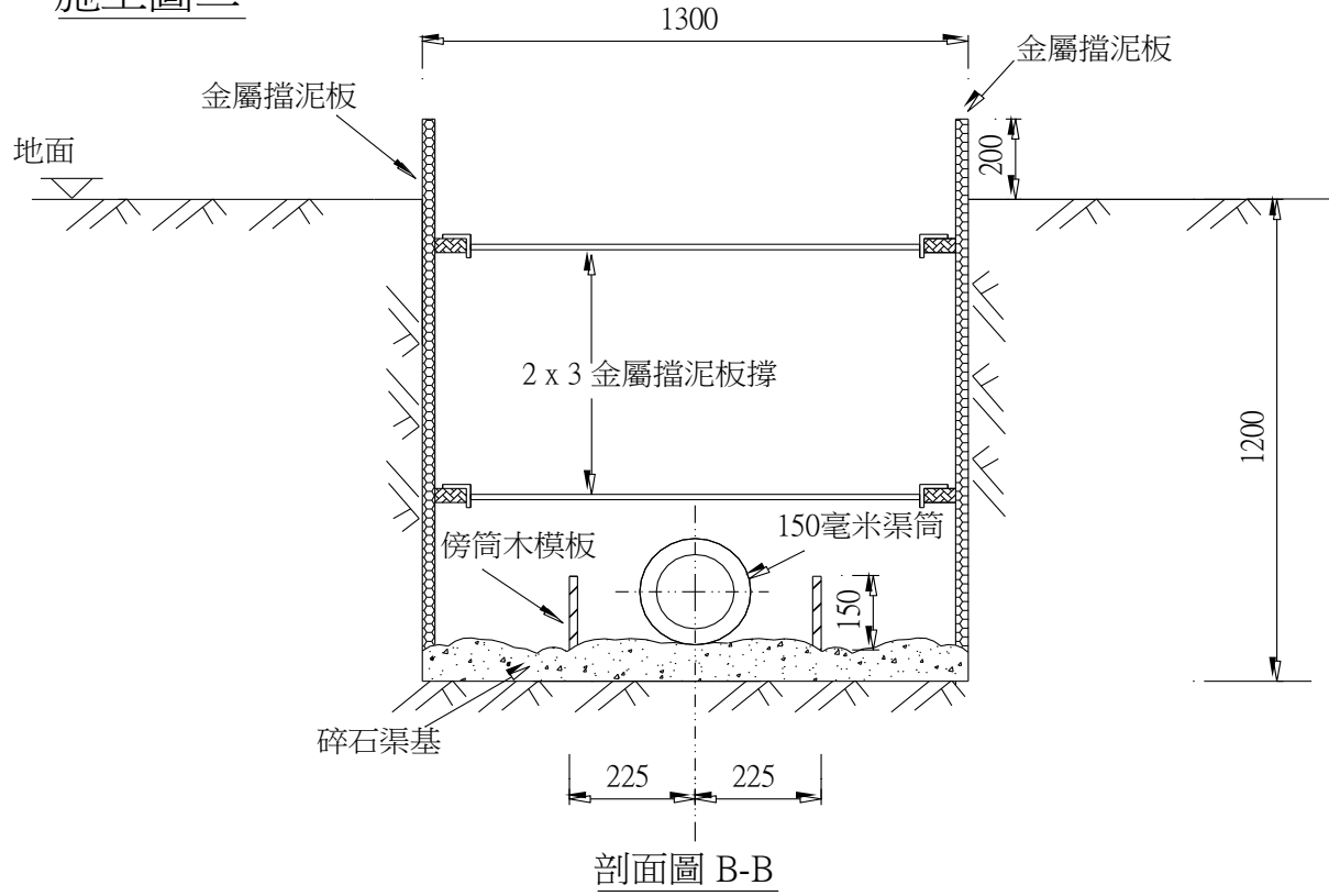
安裝擋泥板、釘製傍筒木模板
