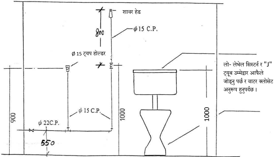
अगाडिको एलिवेशन 'A-A'
