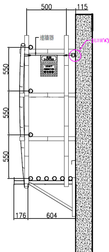
TOS SE3 側面圖C
