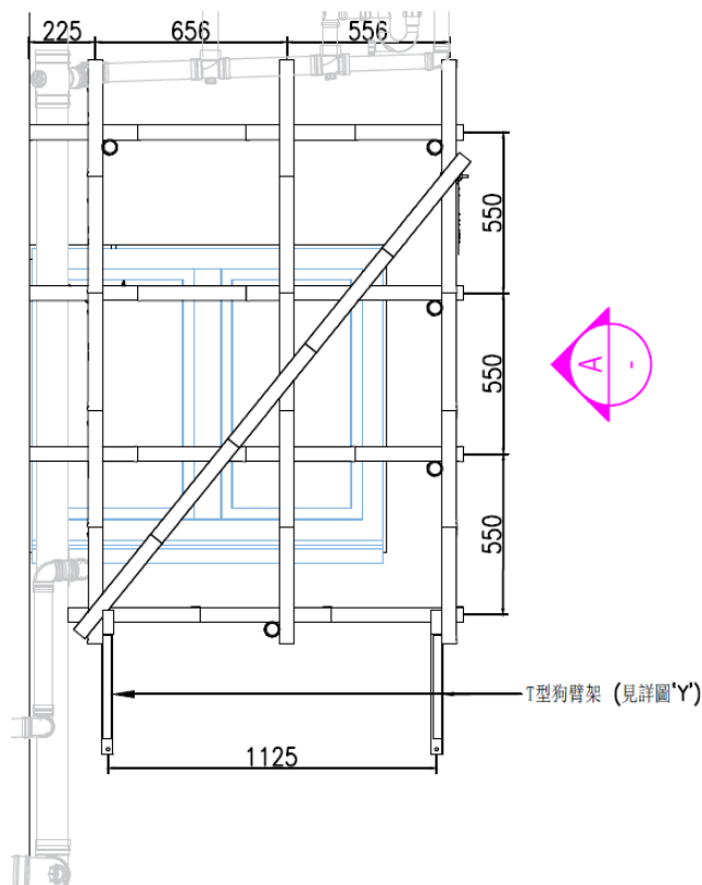
TOS SE1 立面圖1
