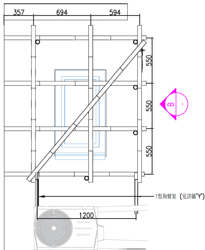
TOS SE2 立面圖2
