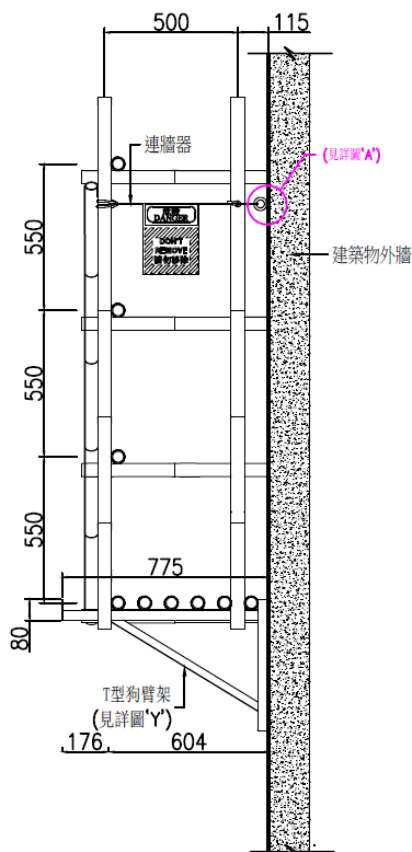
TOS SE1 側面圖A
