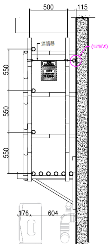
TOS SE2 側面圖B
