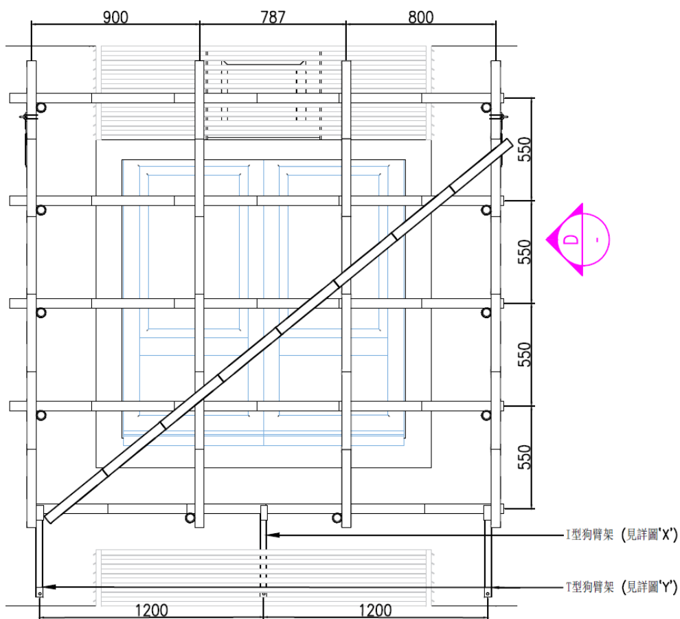
TOS SE4 立面圖4
