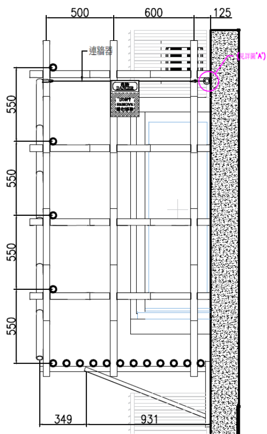
TOS SE5 側面圖E
