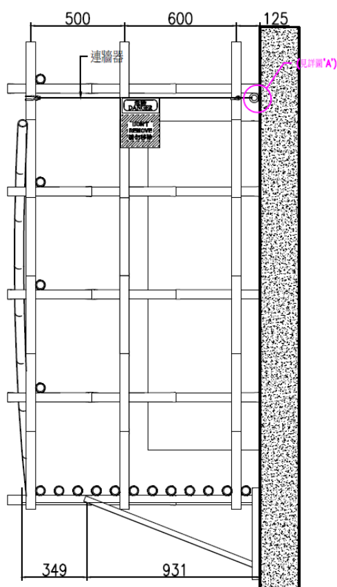
TOS SE4 側面圖D
