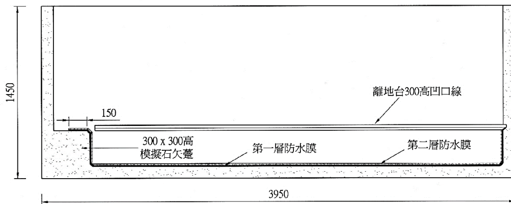
剖面圖 C
