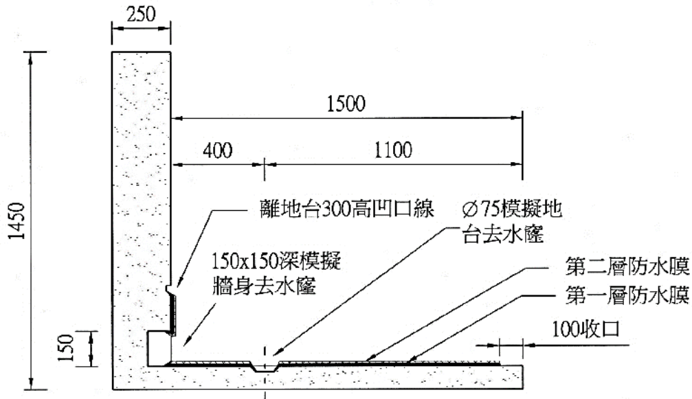
剖面圖 B
