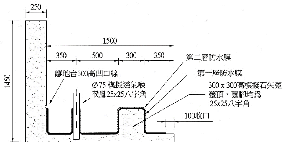
剖面圖 A
