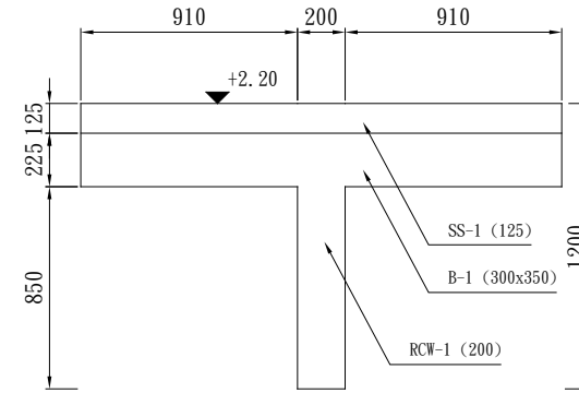
SECTIONAL VIEW B-B सेक्शनल भ्यू B-B
