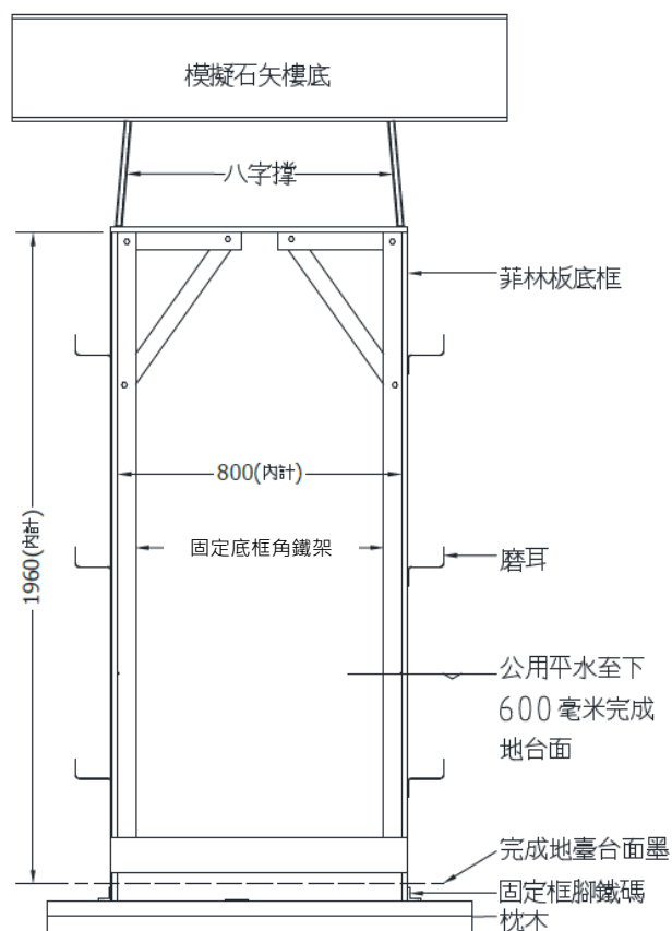
正視圖
