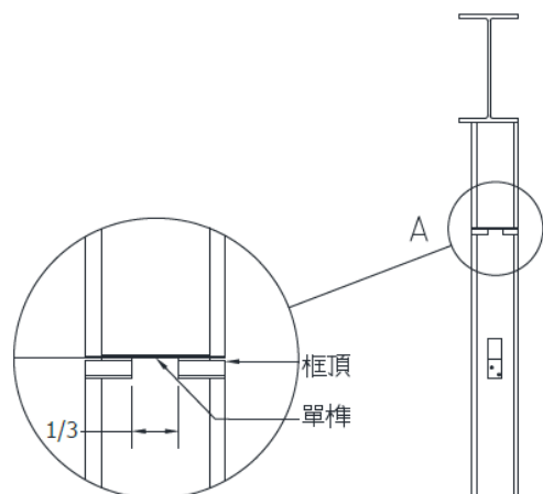
詳細視圖 A
