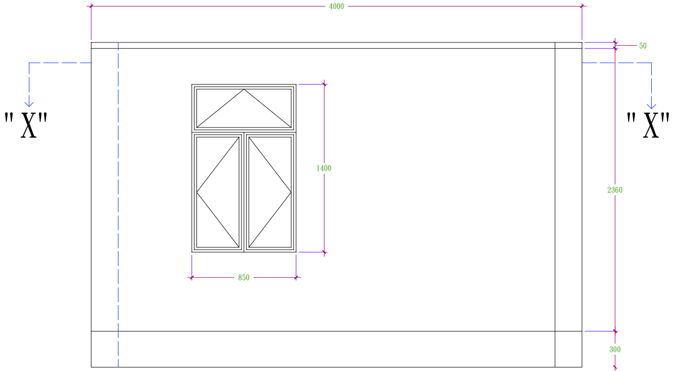
Elevation
