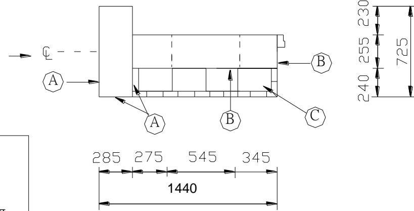
क्षैतिज प्लान
