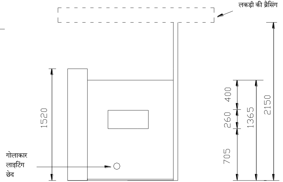
फ्रंट एलिवेशन
