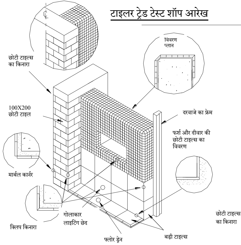
3-D प्लान
