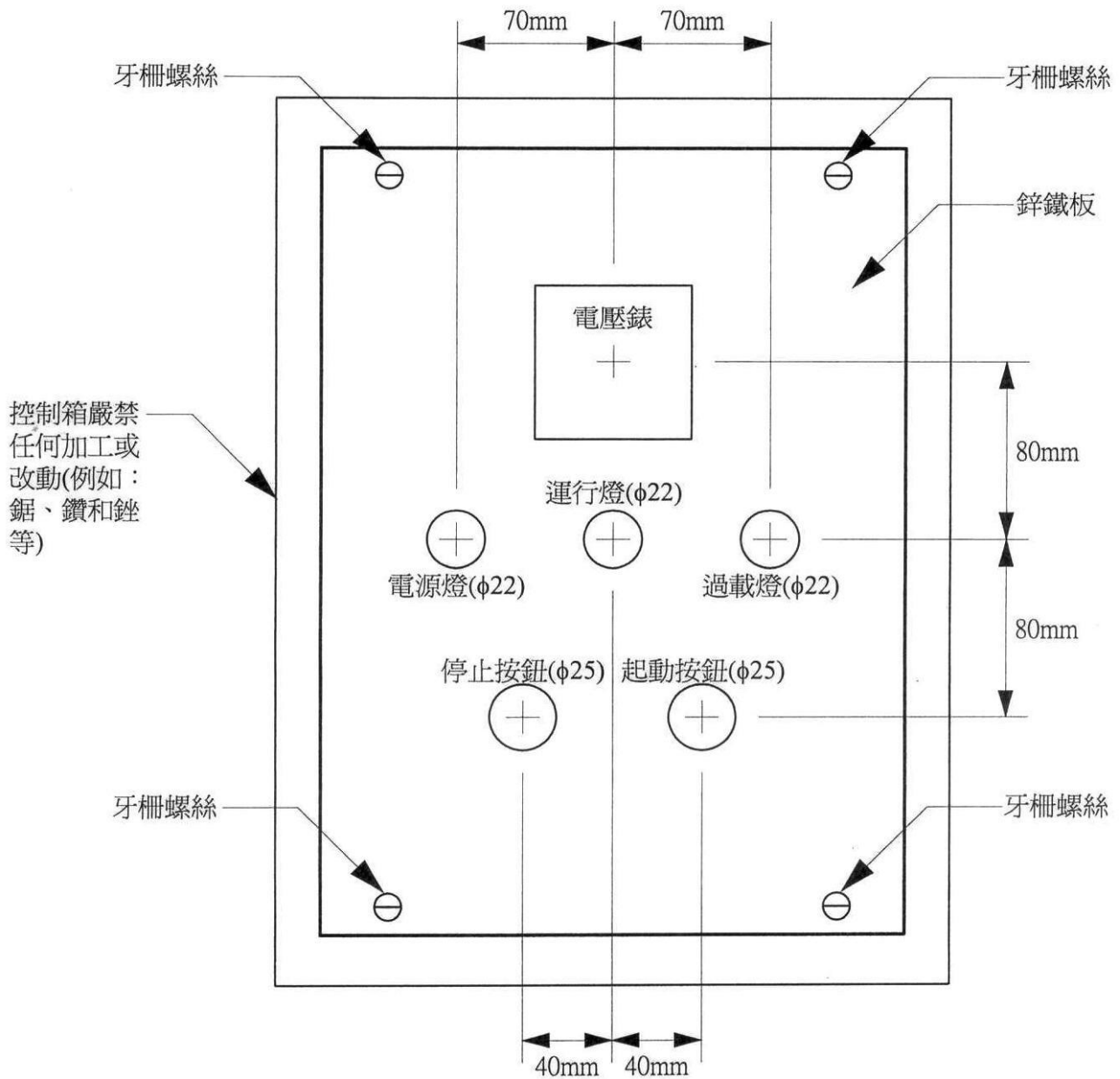
控制板面零件裝配位置
